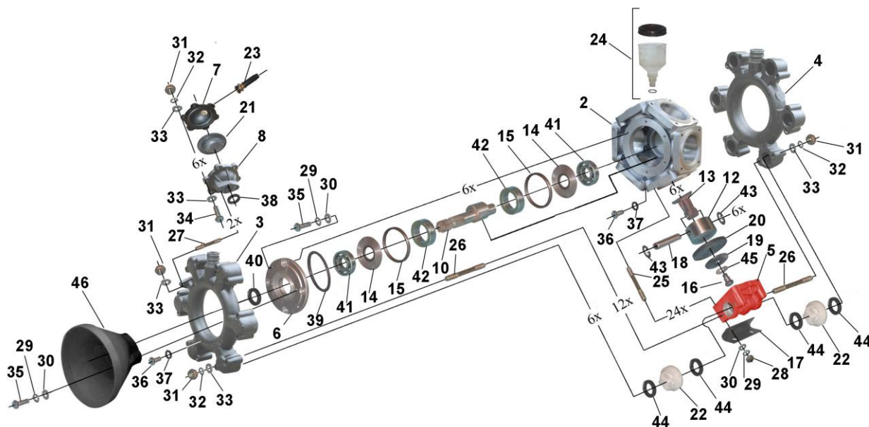
Rys.1 Budowa pompy PPT200
